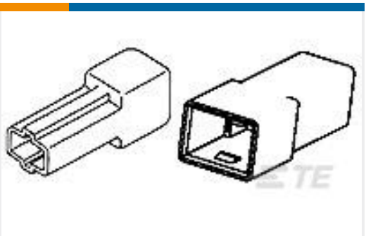
TE 产品编号180916-5 FF 250 TAB HSG 1P NYLON BLACK
