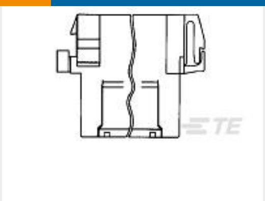
TE 产品编号1-929505-4 TAB HSG .110 (2.8 MM) HSG TAB
