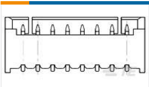
TE 产品编号1-1734829-1 1.25 WTB HDR DIP, 11 POS
