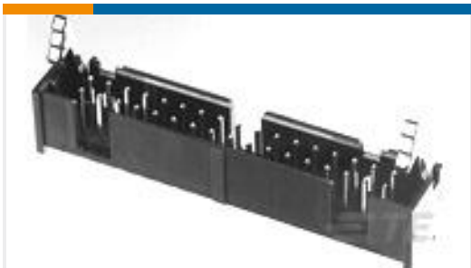
TE 产品编号3-1761608-6 IDC LOW PRO HDR 60P VERT SHT L
