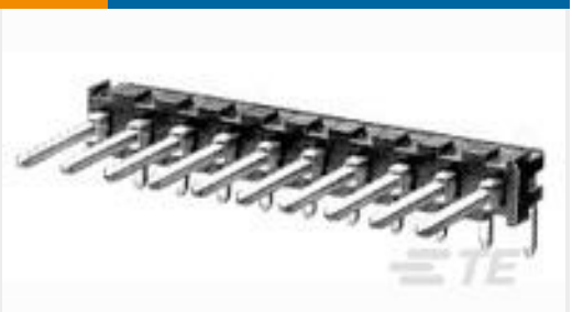
TE 产品编号1-87233-2 12 MODII HDR SRRA UNSHRD .100
