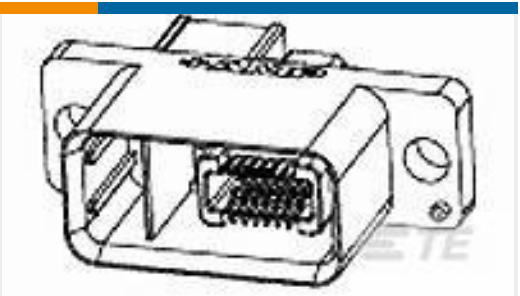
TE 产品编号1-292239-2 1.5 MINI CT HYBRID DRAWER 16P
