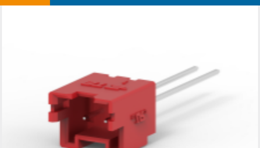
TE 产品编号1-2299683-2 EP2.5 HDR 2P VERT W/O BOSS, TAPING,RED
