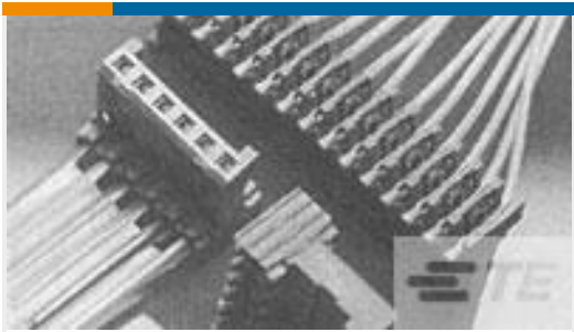
TE 产品编号 144274-8 PLUG HE13 IDC 90 8 P AWG 26
