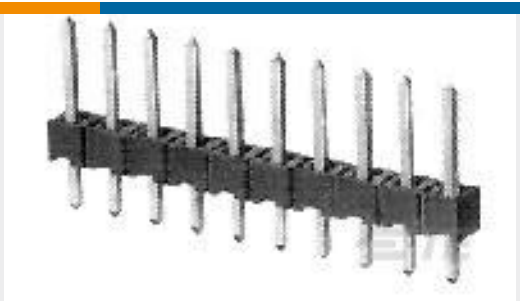
TE 产品编号4-826629-0 40P AMPMODU II STIFT LEI
