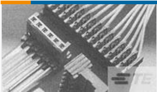
TE 产品编号 1-144270-0 PLUG HE14 IDC 90 10 P AWG 24
