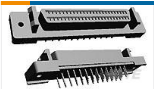
TE 产品编号749721-3 28 50SR VERT RCPT ASSY
