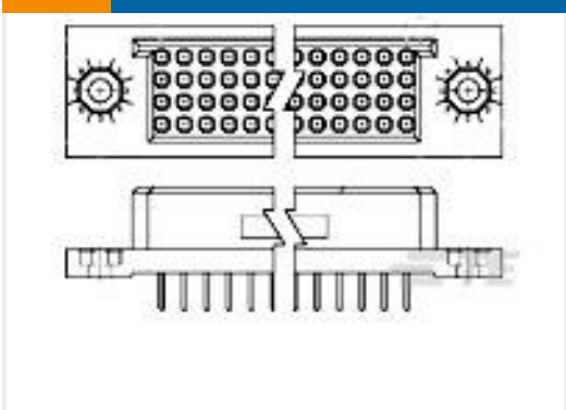
TE 产品编号1-533285-2 BOX II 4 ROW RECP ASSY 300 POS
