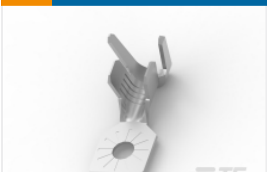
TE 产品编号1544340-1 COSSE PLATE DIA.8,
