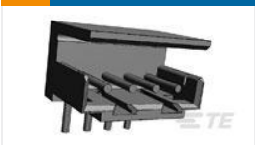
TE 产品编号292250-3 CT P/HDR BOX H ASSY 3P W/KINK
