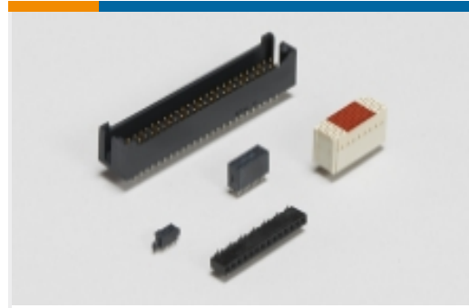
板对板接头和插座(1243)
