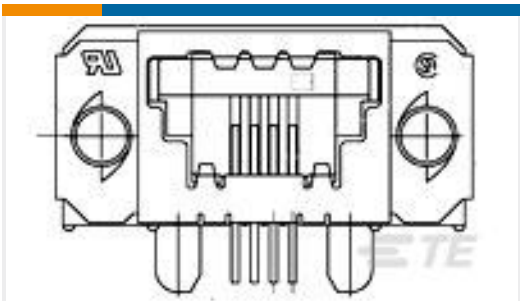
TE 产品编号3-1761185-3 8 SDL SE GRND RCPT ASSY
