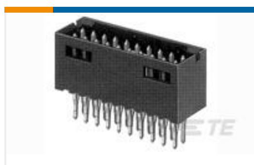
TE 产品编号1-102699-2 26 MODII HDR DRST SHRD A/PIN
