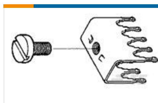
TE 产品编号1-505558-1 10 PWR TAP CONT PLTD MTR .100
