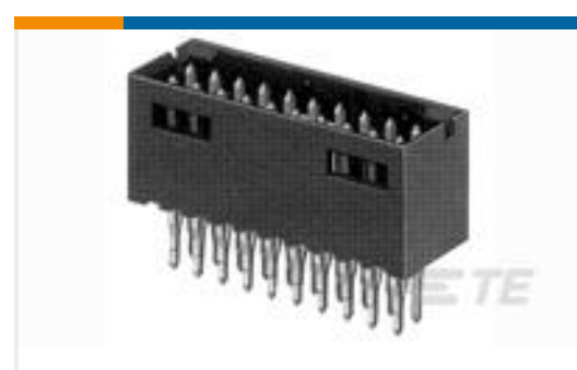
TE 产品编号102699-8 18 MODII HDR DRST SHRD A/PIN
