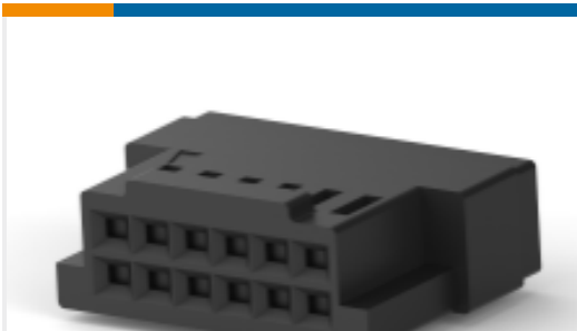
TE 产品编号1-487526-0 2.54mm FFC 连接器母端外壳
