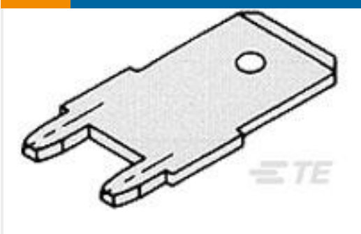
TE 产品编号1217566-1 250 FASTON,PCB TAB,TCBR
