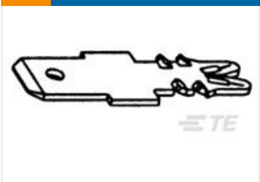
TE 产品编号3-1601174-2 .187 X .032 TAB STD SIAMEZE
