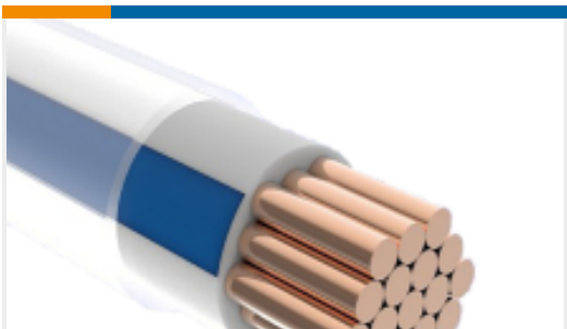
TE 产品编号E816483001 ACW0219-1.00-8(NS)
