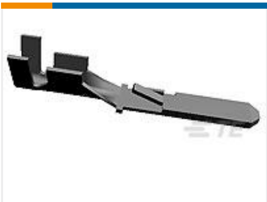
TE 产品编号160743-2 FF 110 TAB 0.5-1.5MM2 PTPBR
