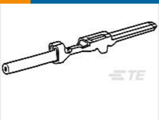
TE 产品编号175208-1 070 TAB CONTACT 16-20
