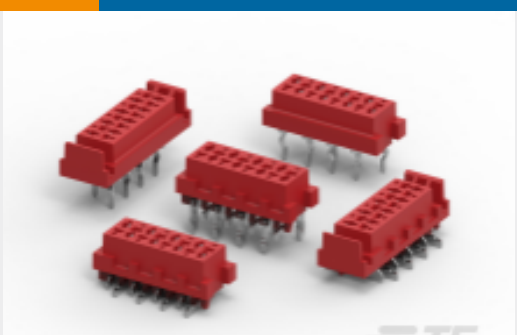
TE 产品编号1-215079-4 板母端连接器顶端插入
