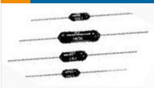
TE 产品编号4-1879645-1 H8 68R1 0.5% 50PPM
