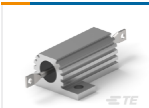
TE 产品编号2-1879071-7 功率电阻器：铝壳体，75 瓦特
