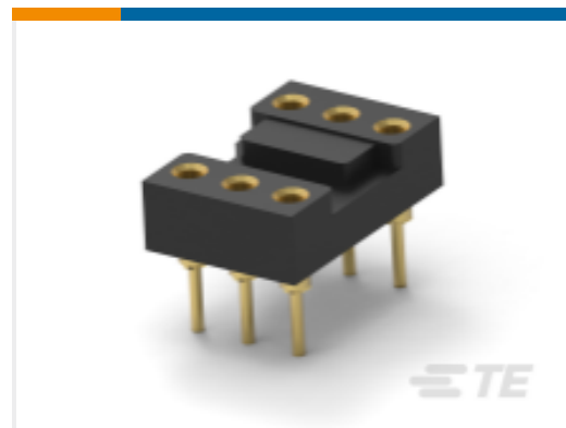
TE 产品编号1-1437535-4 DIP 插座：标准，冲压成型，闭合式，金
