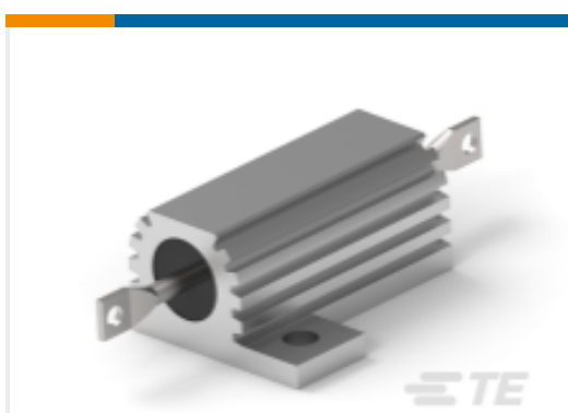
TE 产品编号1879073-7 功率电阻器：铝壳体，75 瓦特
