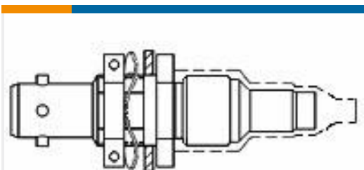
TE 产品编号216081-000 55A0114-26-6
