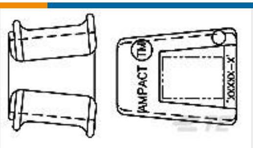
TE 产品编号602380-7 AMPACT Tap 350-350
