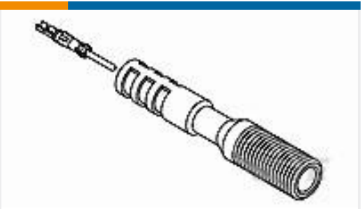
TE 产品编号861753-4 RECEPTACLE ASS'Y
