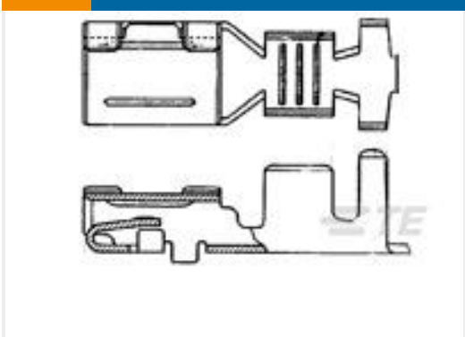
TE 产品编号175042-1 FF 187 REC 2-3MM2 PTBR
