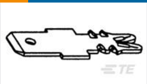
TE 产品编号4-1601035-1 031-081-000=TAB,187X032,STD5MZ
