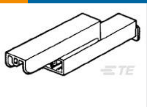
TE 产品编号1-174712-7 PL MKII 187 REC HSG 2P NYLON RED
