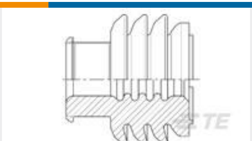
TE 产品编号1355437-3 MCP9,5 EINZELDICHTG
