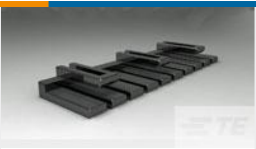
TE 产品编号1-1969443-2 EP 2.5 TPA Retainer, 12 Pos
