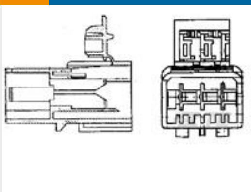
TE 产品编号 1-144836-5 HOUSING TAB 5MM 5 P BROWN
