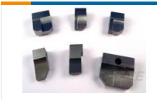
TE 产品编号1-1633927-6 ANVIL
