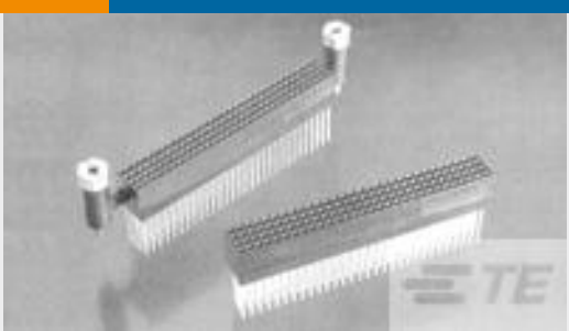
TE 产品编号1375799-3 ASSY, 120 POS PC104 PLUS
