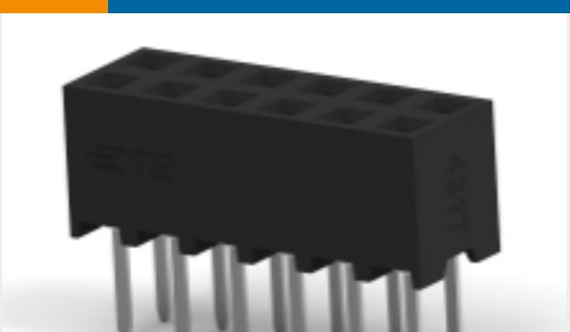
TE 产品编号1-2314812-2 12P, 2MM, B-B, REC, DRVT, 2.0, 0.1AU, TB, W/CAP
