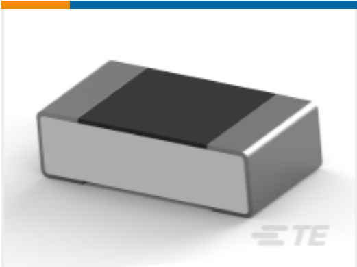
TE 产品编号6-2176367-1 RQ 0603 19K6 0.1% 10PPM 1K RL
