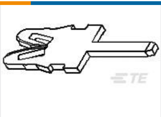
TE 产品编号1601138-1 151-005-000=TAB,3.3X0.8,MEDSMZ
