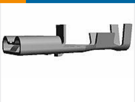
TE 产品编号170329-1 250 PL MKII REC. 15-10AWG PTBR
