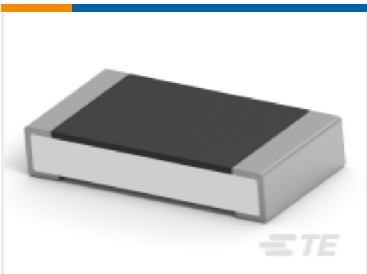
TE 产品编号8-2176390-5 RQ 1206 8K66 0.1% 10PPM 5K RL
