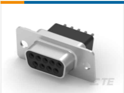
TE 产品编号1-5747150-3 D-Sub 插座组件：垂直，外壳尺寸 1，2.74mm
