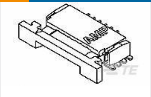
TE 产品编号1-84952-4 1MM FPC HORZ.BTTM CONT.ASS.14P
