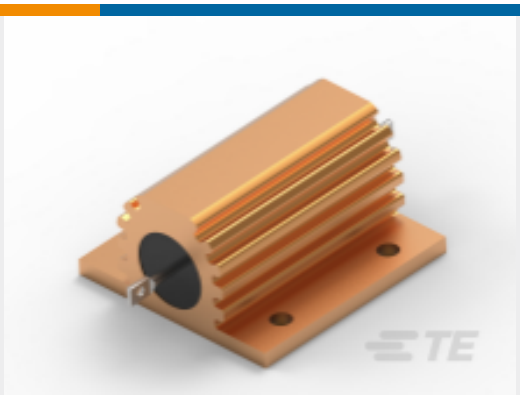
TE 产品编号3-1676625-0 功率电阻器：铝壳体，HSA
