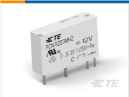
TE 产品编号3-1461491-3 PCN 3A/5A 纤薄 PCB 继电器 12VDC
