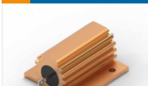
TE 产品编号1676625-3 功率电阻器：铝壳体，HSA
