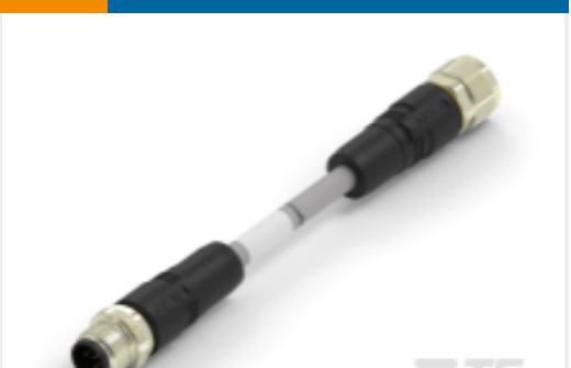
TE 产品编号TAA755A1611-060 现场总线，DeviceNet M12 A 码 5p PVC DE
