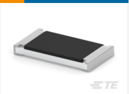
TE 产品编号2-1622824-5 厚膜电阻器：电流感应
