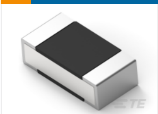
TE 产品编号1-2176304-0 RP 1E 0.1W 12R4 0.1% 25PPM 5K RL
